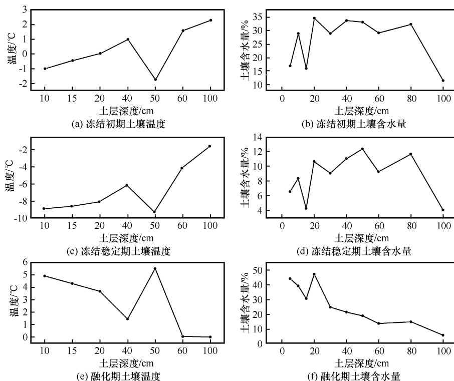
图4 不同冻融阶段的土壤温度与含水量剖面
