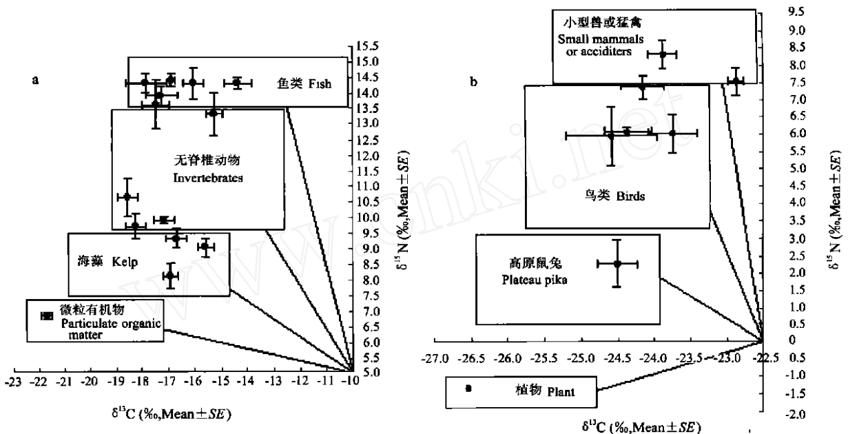
图 4 海洋生态系统 (a) 和高寒草甸生态系统 (b) 的稳定性同位素碳 ( ^{13}\text{C} ) 和氮 ( ^{15}\text{N} )
