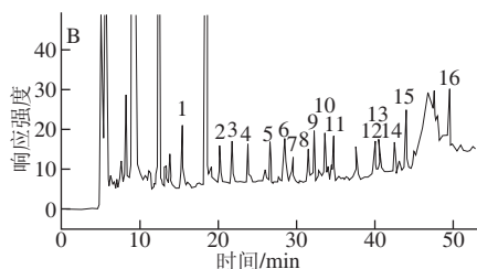
1.醋酐; 2.磺胺噻唑; 3.磺胺吡啶; 4.磺胺甲基噻唑; 5.磺胺二甲恶唑; 6.磺胺二甲噻唑; 7.磺胺甲氧吡嗪; 8.磺胺氯吡嗪; 9.磺胺甲恶唑; 10.磺胺间甲氧吡嗪钠; 11.磺胺二甲异恶唑; 12.磺胺苯吡唑; 13.磺胺氯吡嗪钠; 14.磺胺间二甲氧吡嗪; 15.磺胺喹恶啉; 16.磺胺硝苯。A.空白鸡肉样品; B.加标样品。
